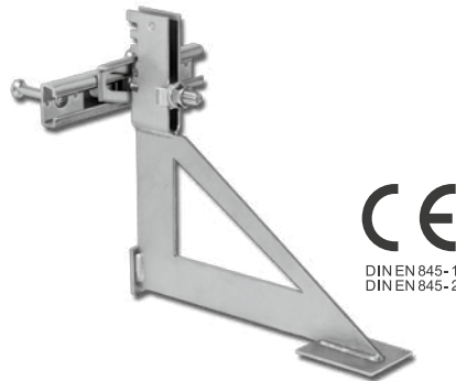
HALFEN HK4 Konsolanker für Verblendmauerwerk
