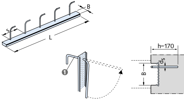
① Standardbügel Typ 1
