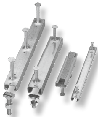
Eine Auswahl des Halfenschienen-Sortiments
