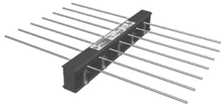
HALFEN HIT-HP/-SP Balkonanschluss
