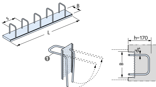
① Standardbügel Typ 5
