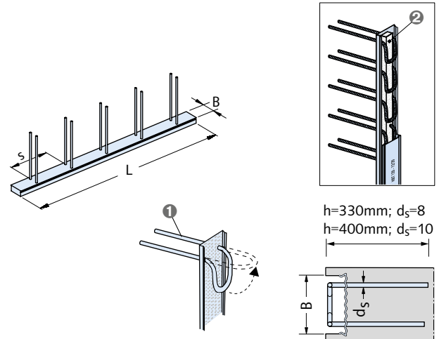
① Standardbügel Typ 6
