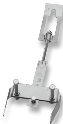
HALFEN Fassadenplattenanker FPA für Beton-Fertigteilfassaden
