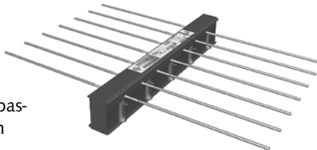
HALFEN HIT-HP/-SP MV Balkonanschluss
